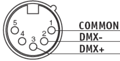
Şekil 3.1: 5 pinli jak
