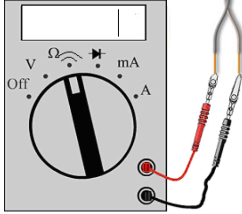
Şekil 2.4 : Kablo kısa devre testi
