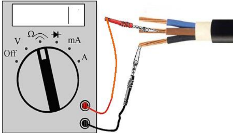
Şekil 2.3: Kabloda açık devre testi
